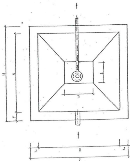
ΚΑΤΟΠΗ
